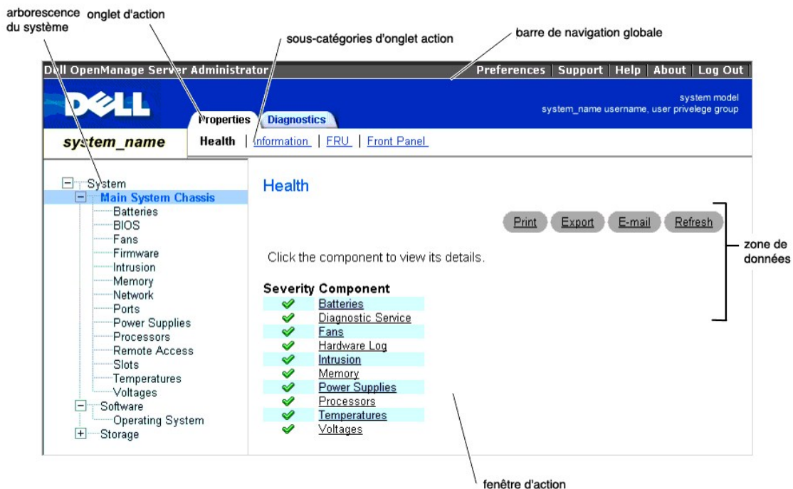
Figure 6-1. Exemple de page d'accueil de Server Administrator
